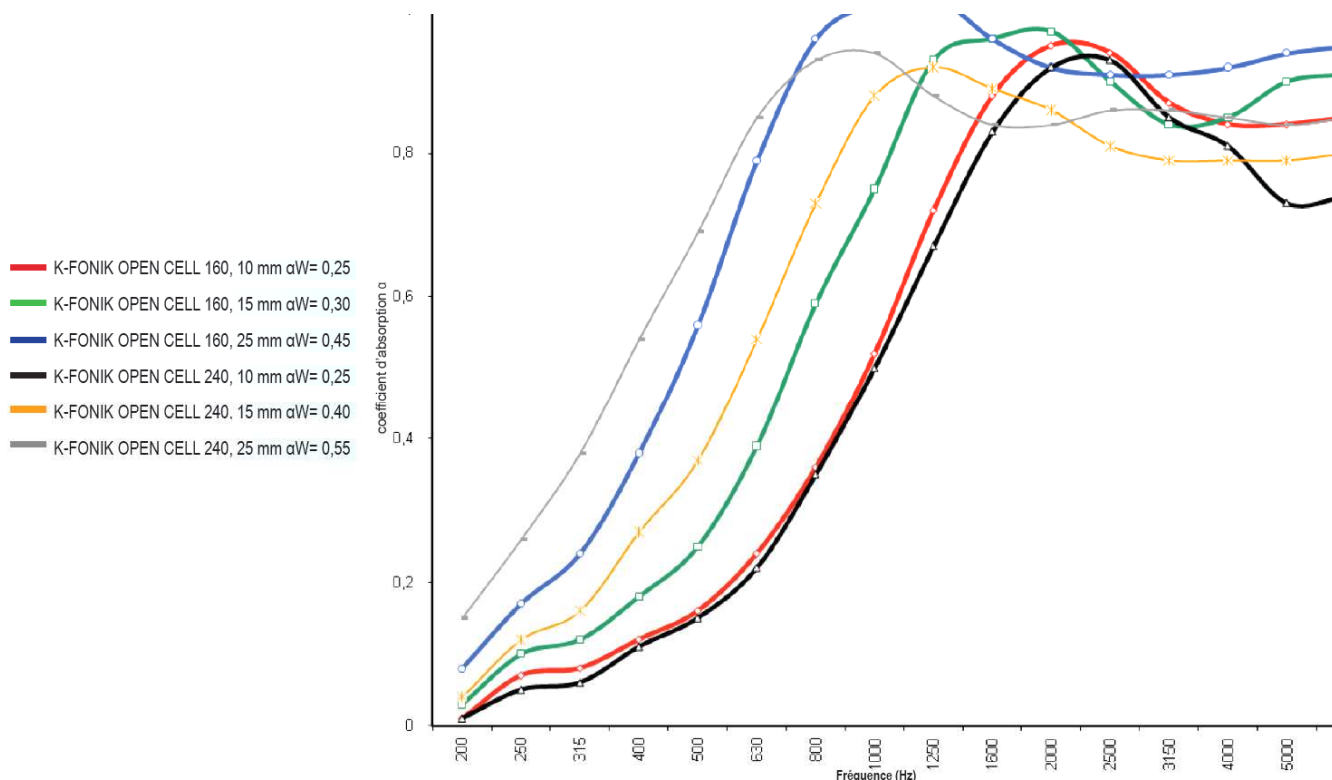
Coefficient d'absorption \alpha_{\text{sabine}} selon UNI EN ISO 354:2003 - UNI EN ISO 11654:1998
